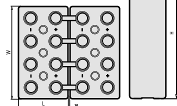
Fig. F Type OPzV
