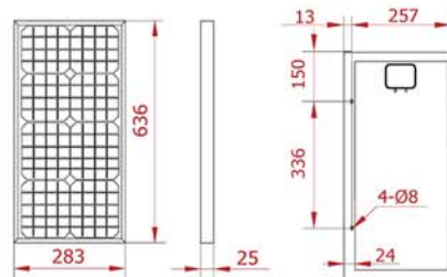
DIMENSIONES/DIMENSIONS ESF-20MA ESF-20PA
