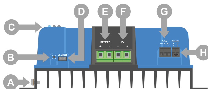
Modèle Tr.
