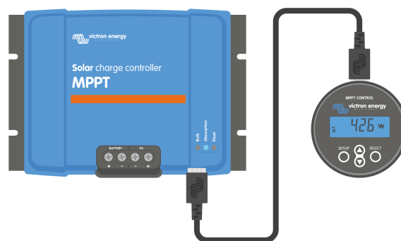
Raccordez l'écran au chargeur solaire en utilisant un câble VE.Direct.
