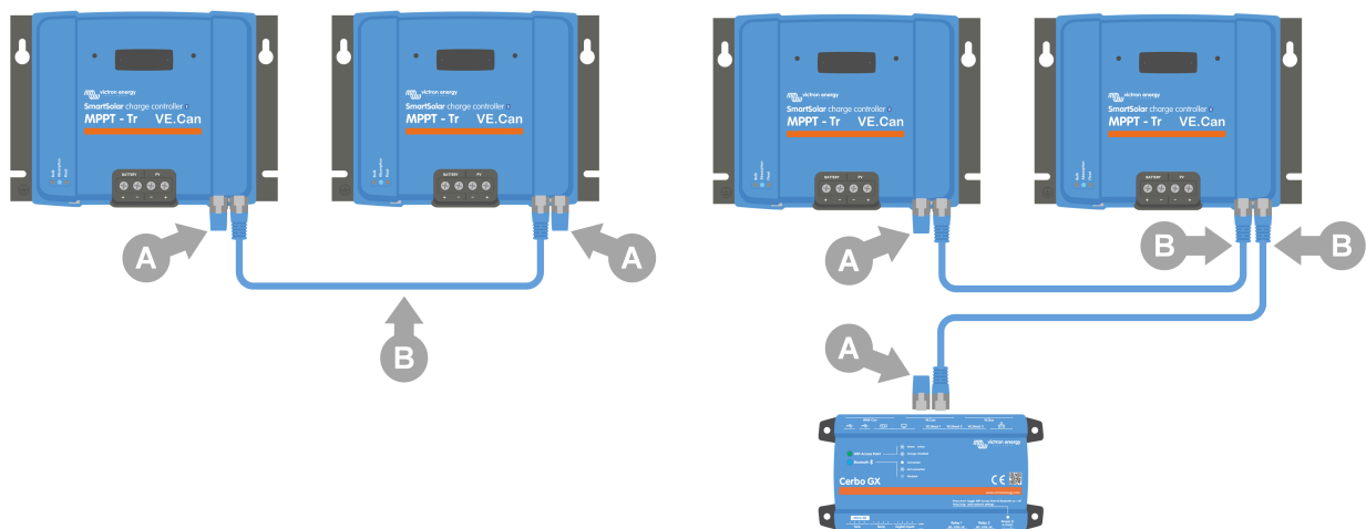
R : Terminaison VE.Can - B : Câble RJ45 UTP.
